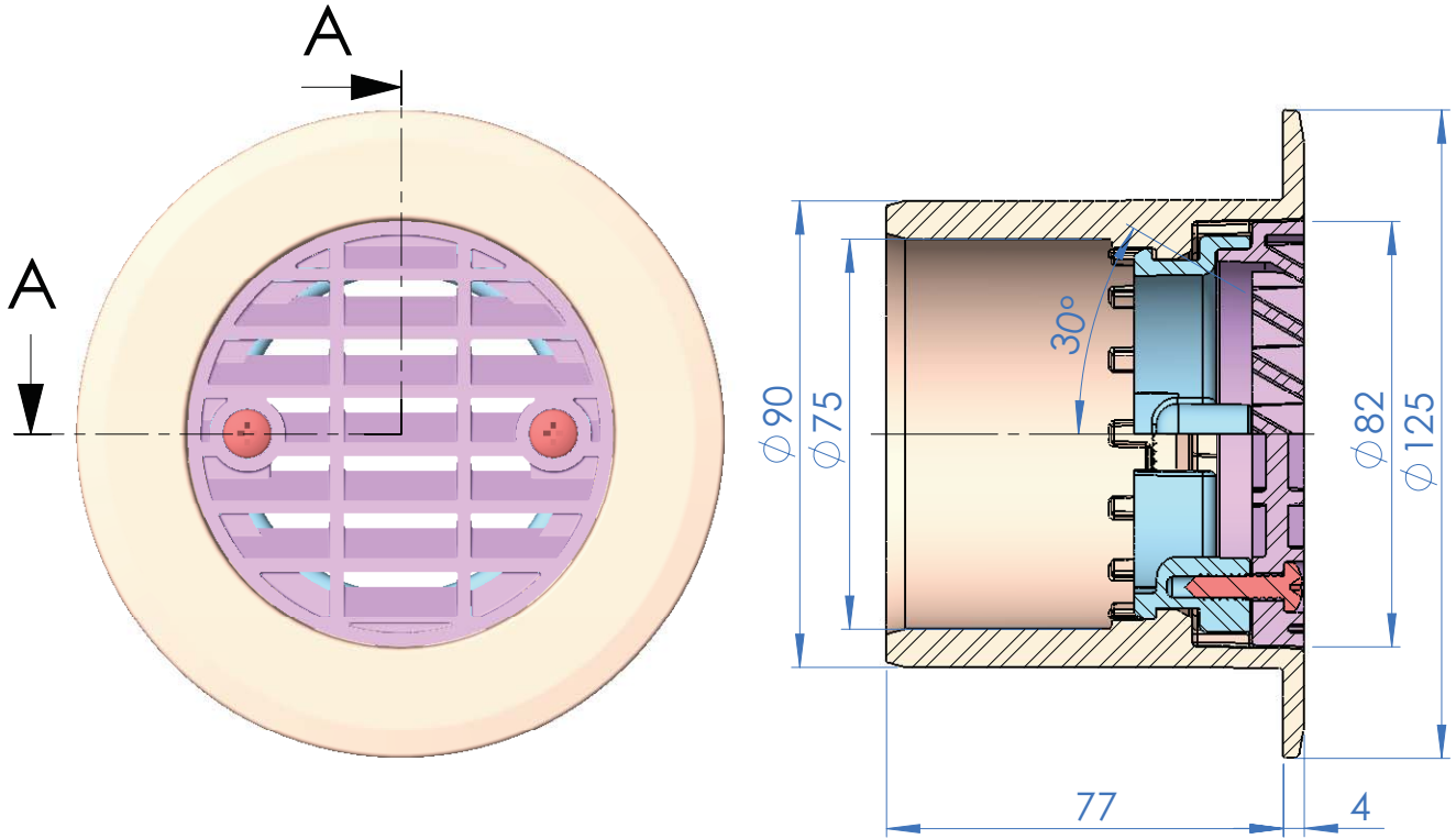
SECCIÓN A-A
