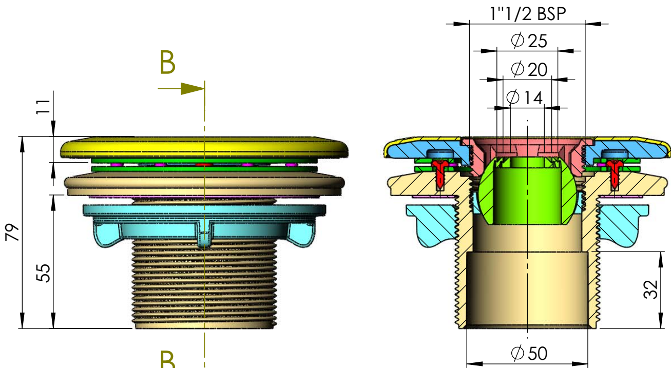
SECCIÓN B-B
