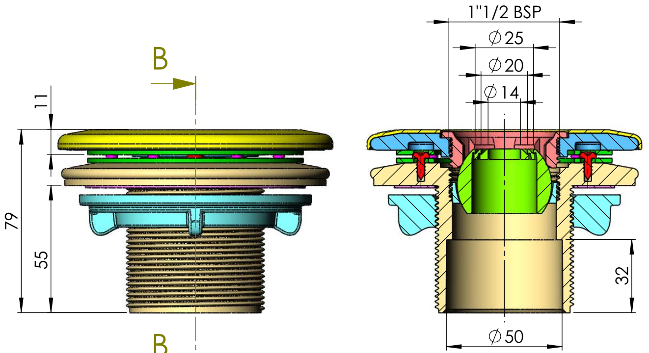
SECCIÓN B-B
